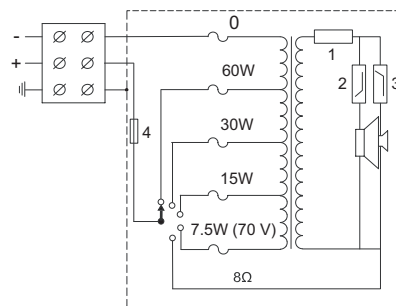
Schéma zapojení (1: pasivní omezovač, 2: dolní propust, 3: horní propust, 4: tepelná pojistka)
